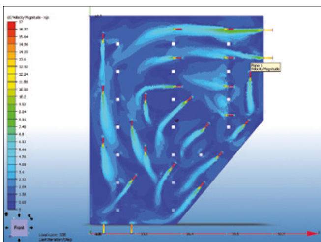
Přodorysné rozložení JET FAN
