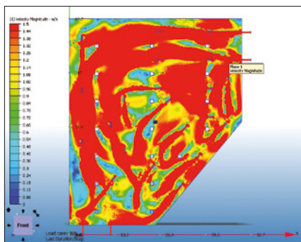
Rychlostní pole JET FAN
