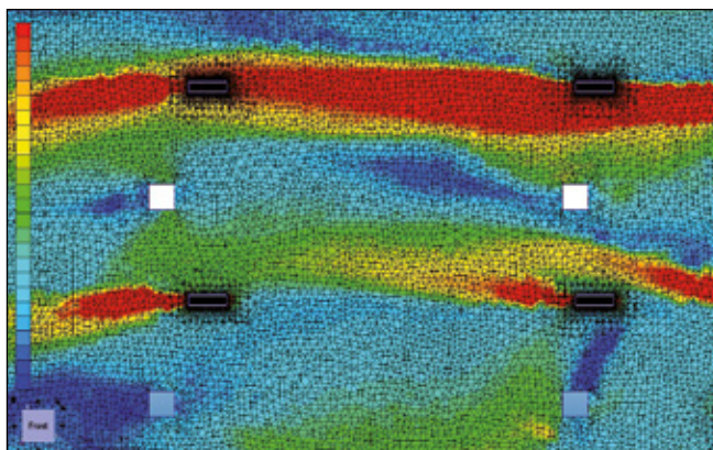
Přodorys rychlostního pole
