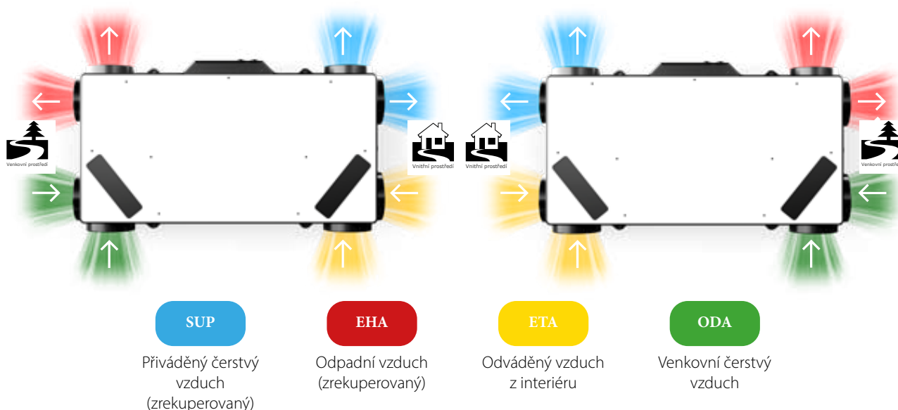
Levé provedení
