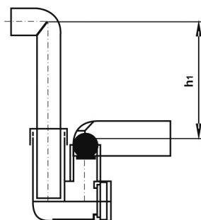
Kuličkový sifon
