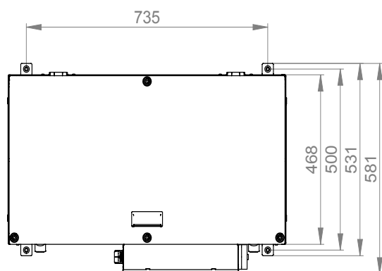
AHAL4-05-VV (vodní výměník)
