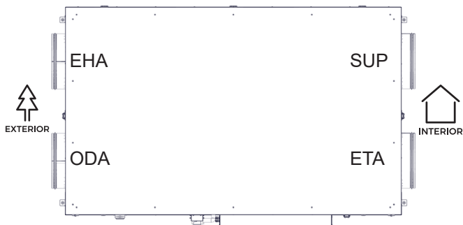
PRAVÉ PROVEDENÍ Pohled shora
