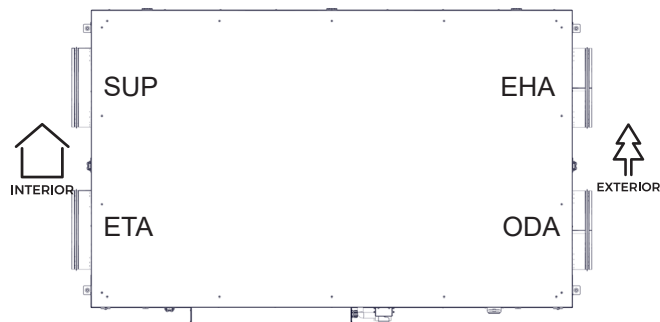
LEVÉ PROVEDENÍ Pohled shora
