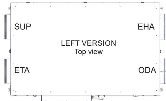
LEVÉ PROVEDENÍ Pohled shora
