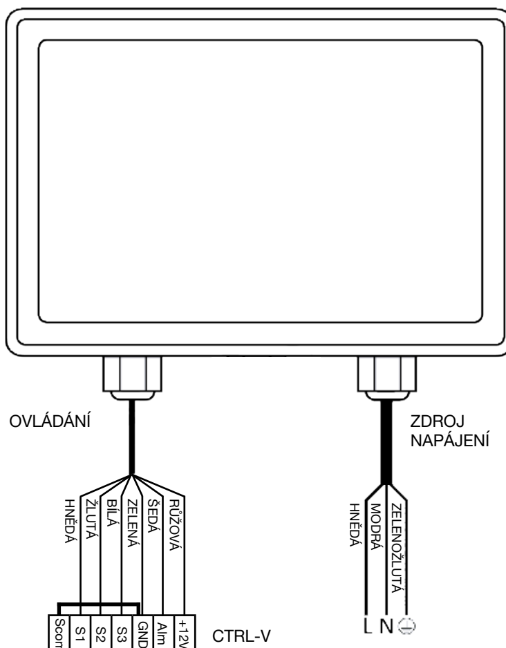
Obr.5.i Elektrické zapojení
