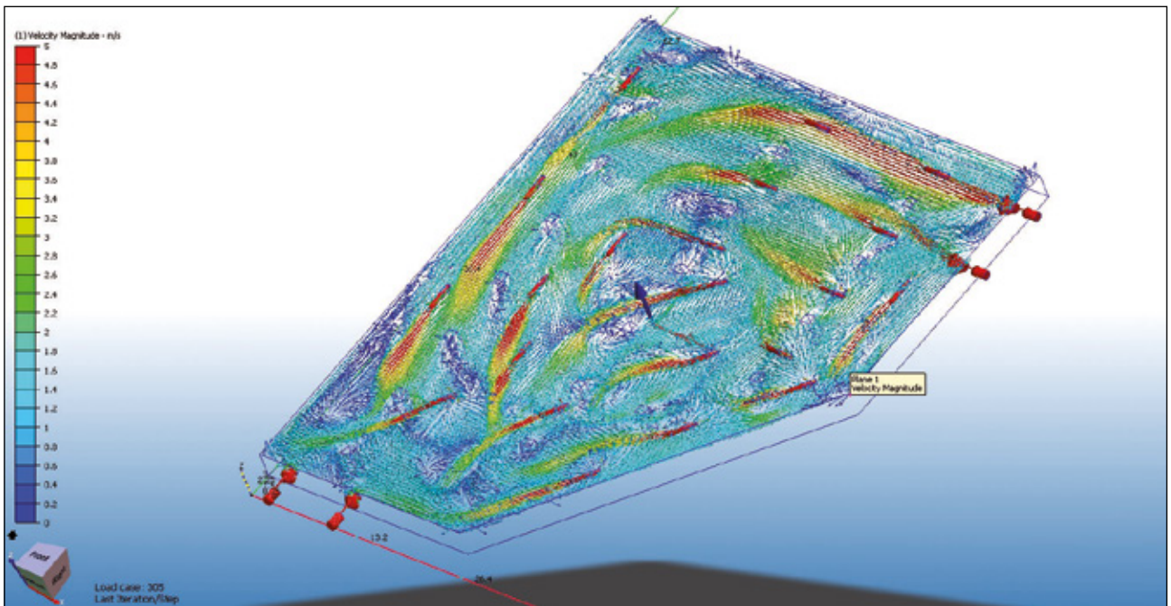
Axonometrie rychlostního pole
