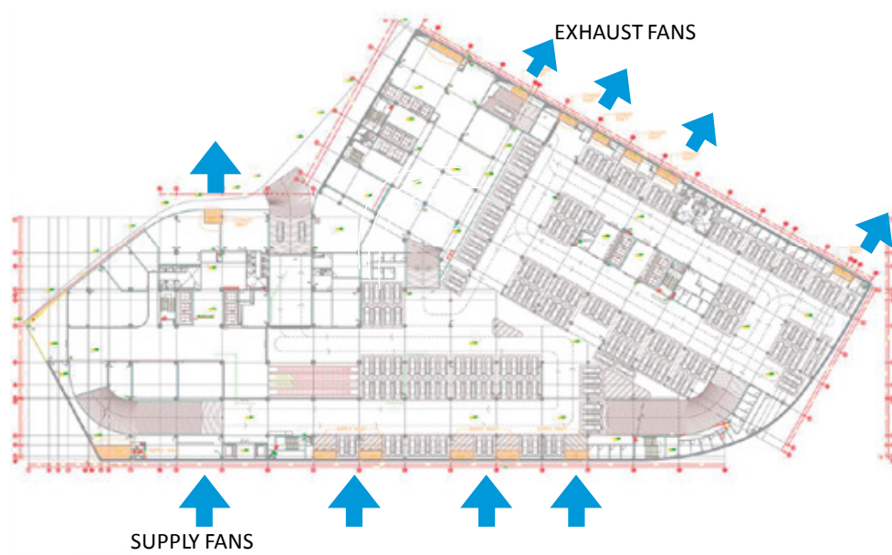
Dispozice garáže s vyznačeným umístěním přívodu a odvodu vzduchu
