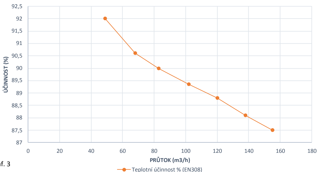
TEPLOTNÍ A VLHKOSTNÍ ÚČINNOST – ERV – MV-XFER-15-20 nominální průtok 150 m 3 /h
